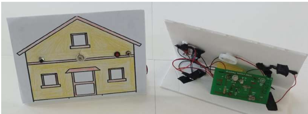
Επίλυση προβλήματος ελέγχου, με κατασκευή ηλεκτρονικού κυκλώματος σε πλακέτα τυπωμένου κυκλώματος και εφαρμογή της σε μοντέλο
