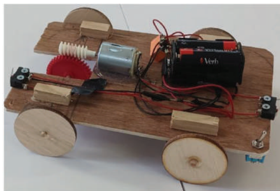
Κατασκευή Οχήματος με μηχανισμό κίνησης ατέρμονα κοχλία συνεργαζόμενου με οδοντοτροχό και χρήση ηλεκτρικού κυκλώματος με ηλεκτρονόμο
